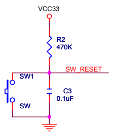
RESET
