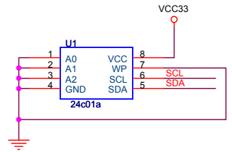
EEPROM
